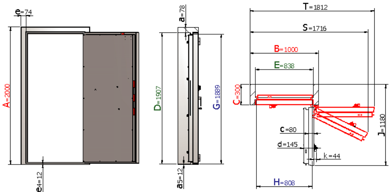
Frontalansicht
