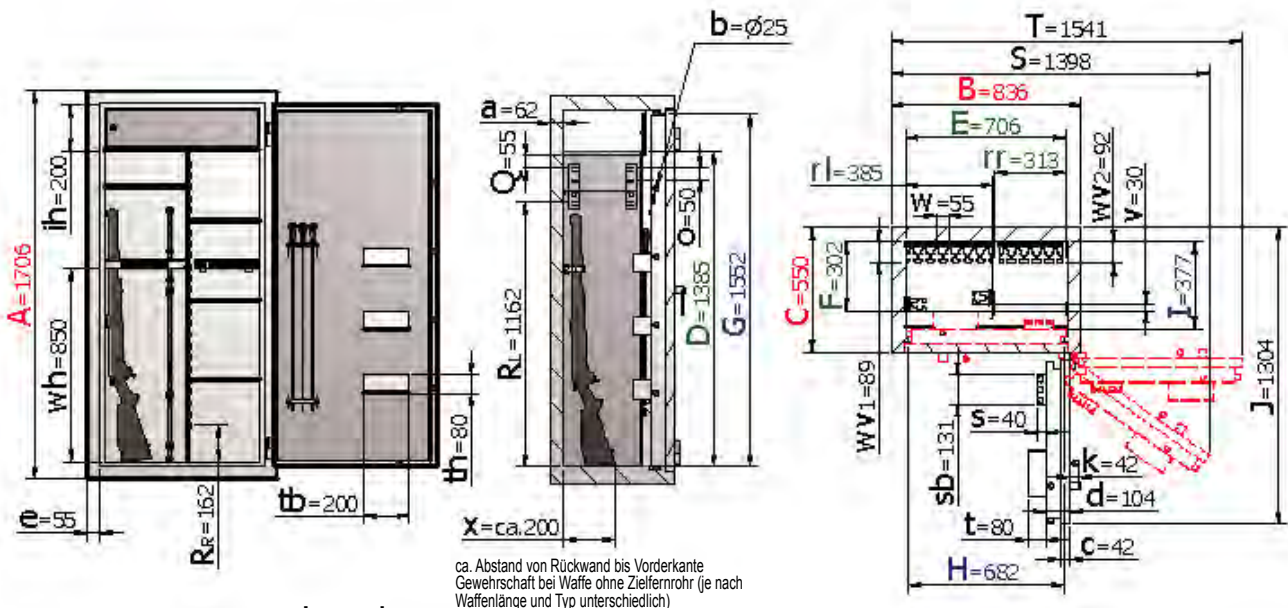
Frontalansicht
