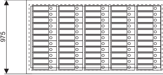
Art. 43106-43108 55 Ordner 75mm (5 Reihen)
