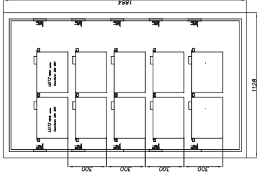
Art. 43109-43110 als Sonderausführung auch 6 Reihen
