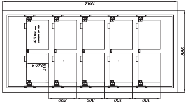
Art. 43104-43105 als Sonderausführung auch 6 Reihen
