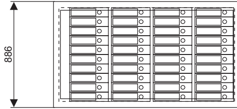
Art. 43100-43101 40 Ordner 75mm (4 Reihen)
