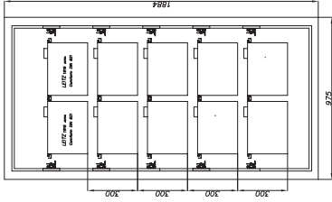
Art. 43106-43108 als Sonderausführung auch 6 Reihen
