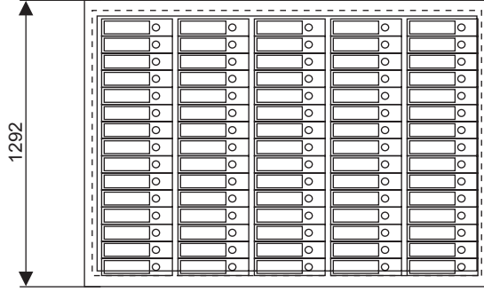
Art. 43112-43114 75 Ordner 75 mm (5 Reihen)
