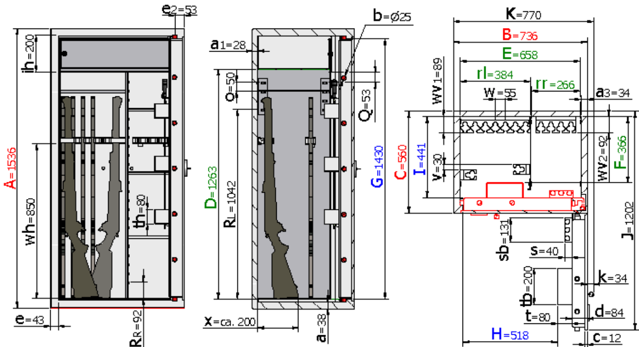
Frontalansicht
