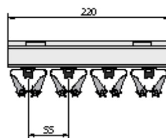
Seitenansicht
