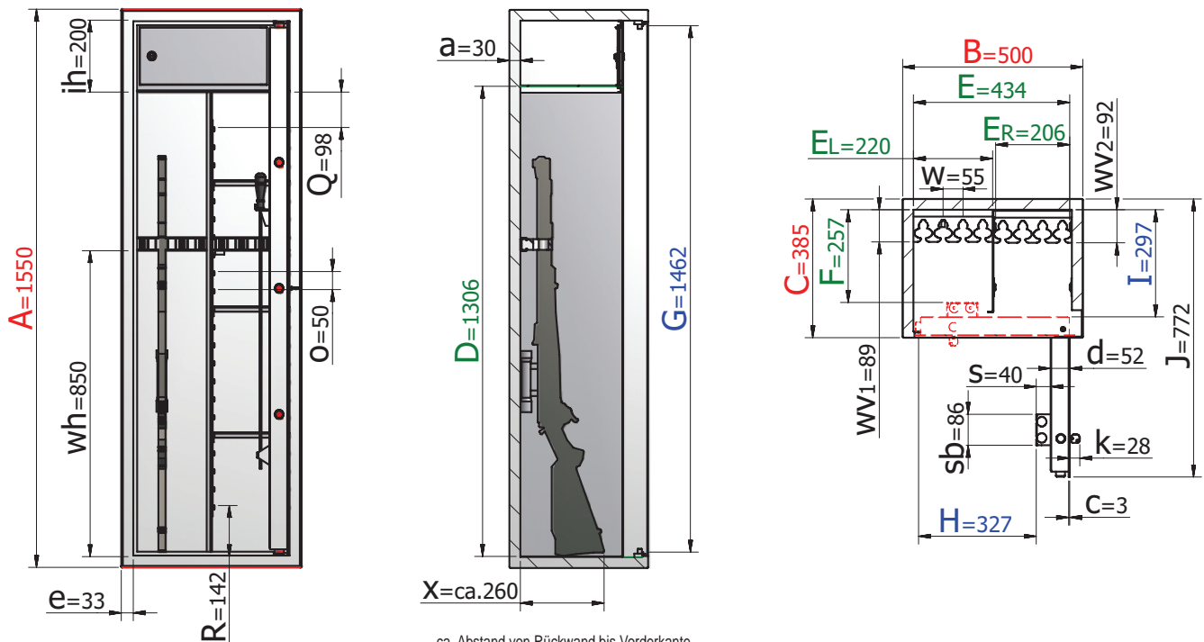
Frontalansicht
