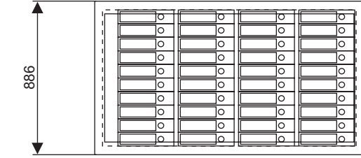
Art. 44600-44601 40 Ordner 75mm (4 Reihen)
